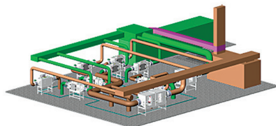
模式实验室内部布局：高效过滤单元、通风管道、送排风机组、化淋配液系统等
